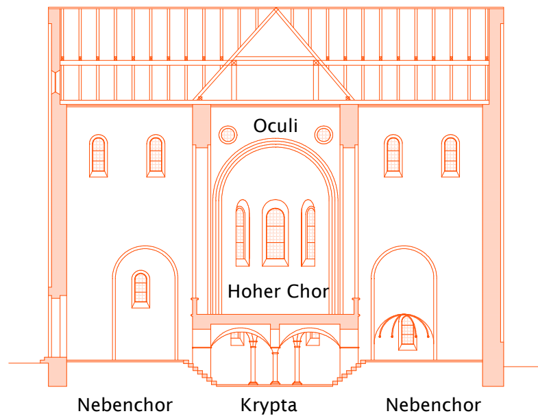
Ansicht Fenster in der Ostwand
